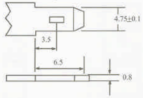
F1 (Fasten Tab No.187E) Standard Terminal
