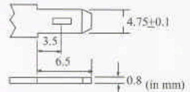
Standard Terminal F1 (Fasten Tab No.187E)
